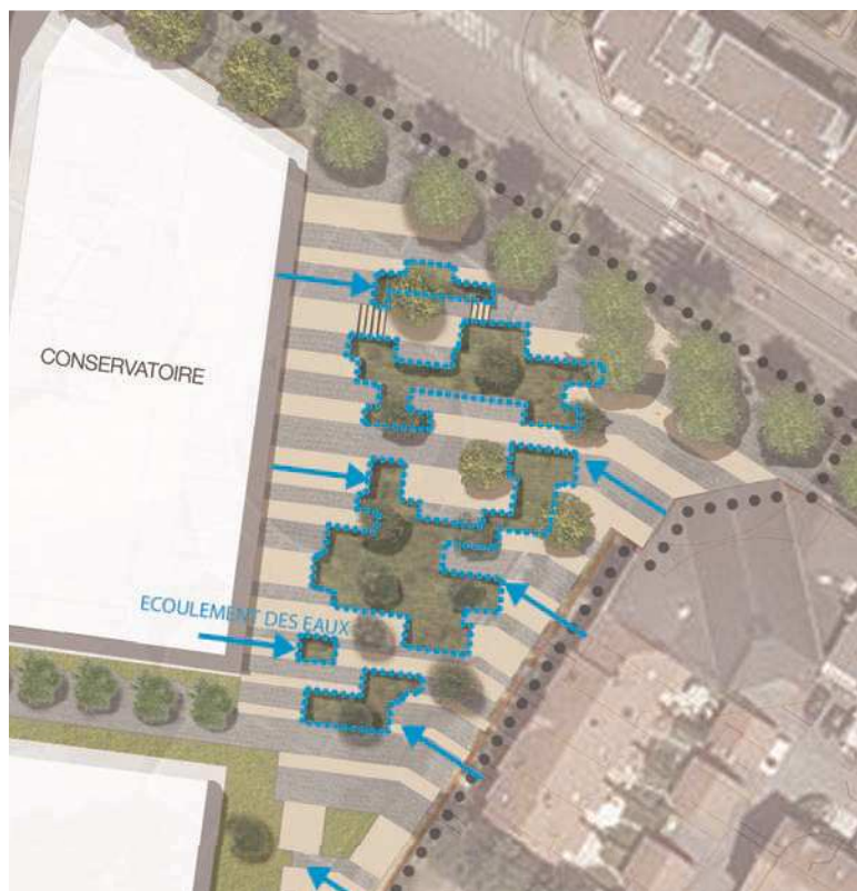
Principe d'infiltration des eaux pluviales dans les jardins en creux
